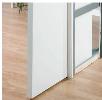
96 mm regelparti för infälld skjuddörr med regelkonstruktion i trä och stål.
