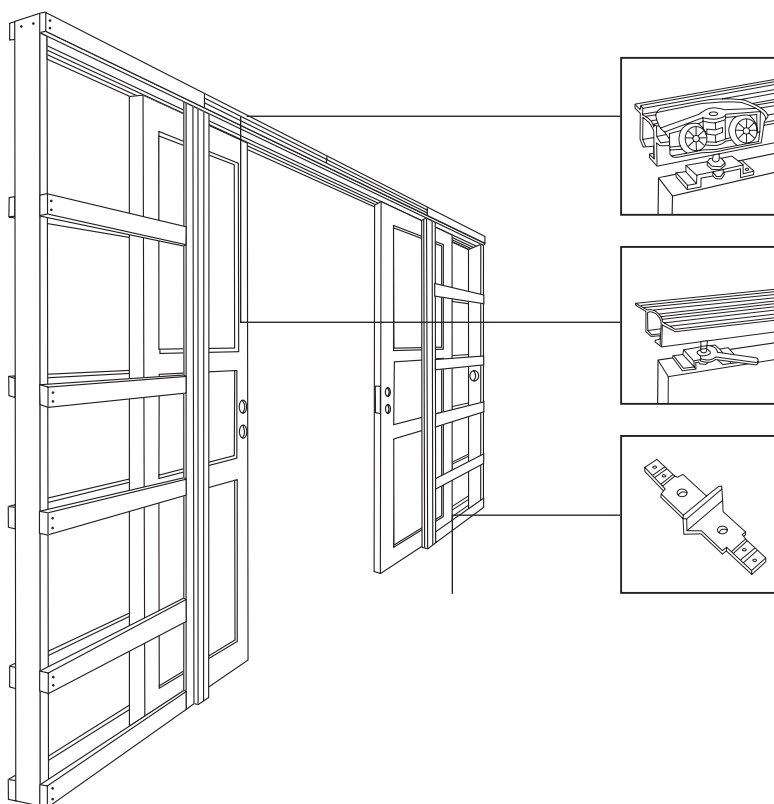
96 mm regelparti för infälld skjuddörr med regelkonstruktion i trä och stål.
