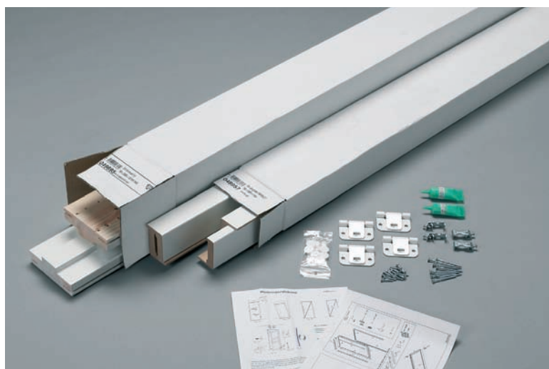
Flexkarmen levereras med hörnbeslag, lim, silikon, skruvar och plastproppar
